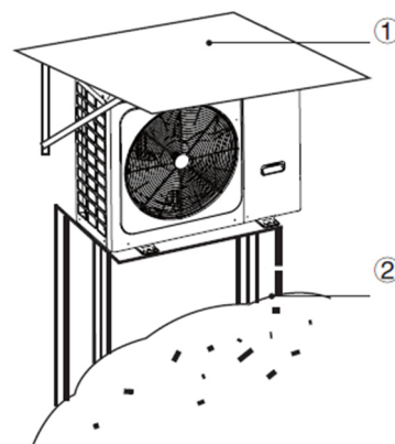
1 - stříška proti sněhu 2 - konzole, podstava
