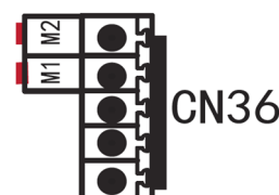
Port CN36 na radiacej doske hydromodulu
