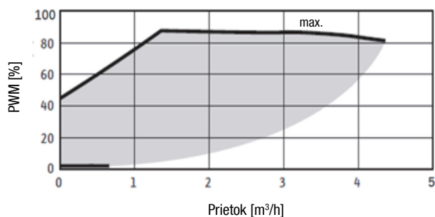
Závislosť medzi PWM a prietokom:
