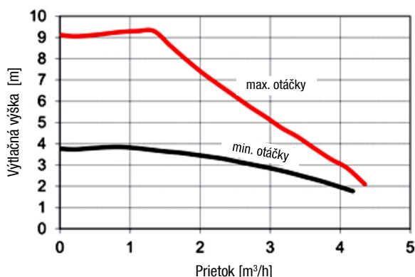
Závislosť medzi výtlakovou výškou a prietokom (regulačný rozsah je medzi krivkou min. a max. otáčok):
