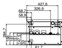
POHĽAD ZOSPODU
