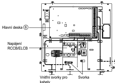
Jak vést volitelné kabely a připojit napájecí kabel (pohled bez interní elektrické instalace)
