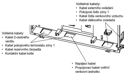
Jak vést volitelné kabely a připojit napájecí kabel (pohled bez interní elektrické instalace)
