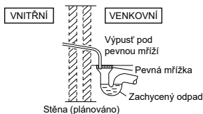
Schéma vypouštěcí hadice do venkovního prostředí.
