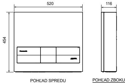
POHĽAD SPREDU
