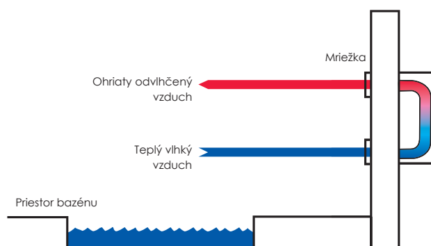
CDP 40T/50T/70T Inštalácia do príslušnej miestnosti s prepojením pomocou potrubnej sady a mriežok (pre steny od 70 do 366mm).
